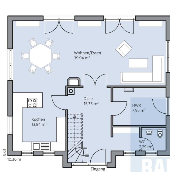
Haus Brede Grundriss
